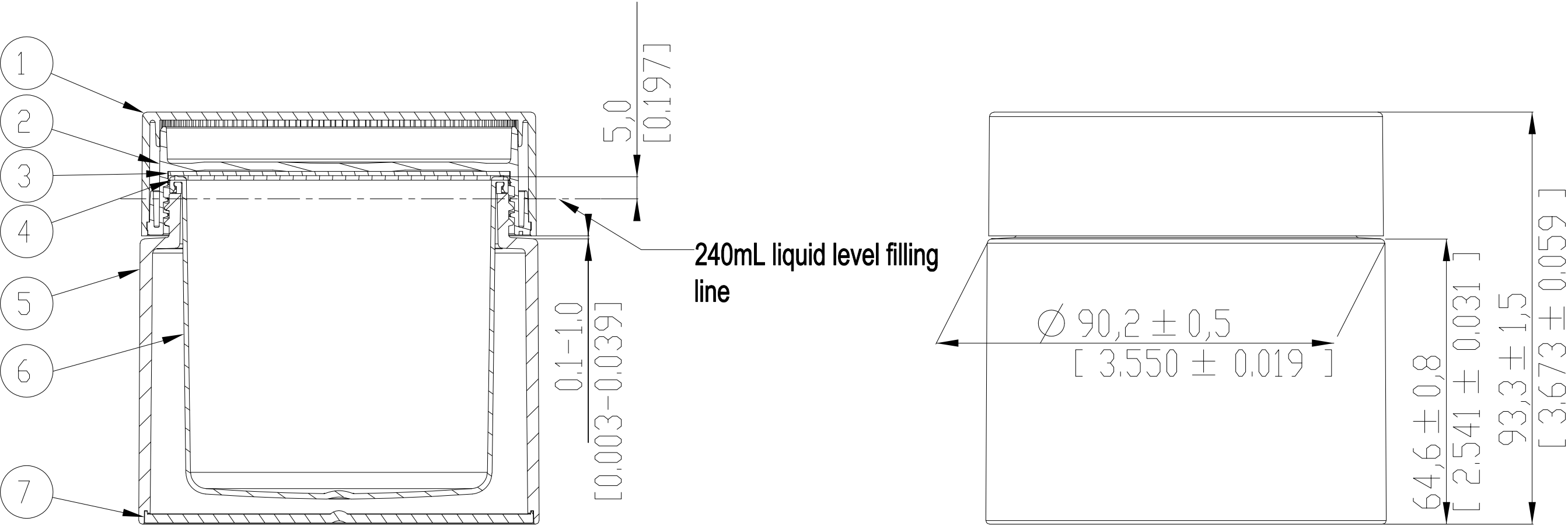
Section A-A
