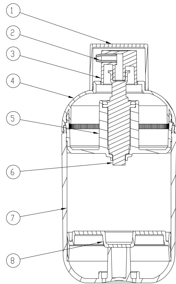
Section A-A
